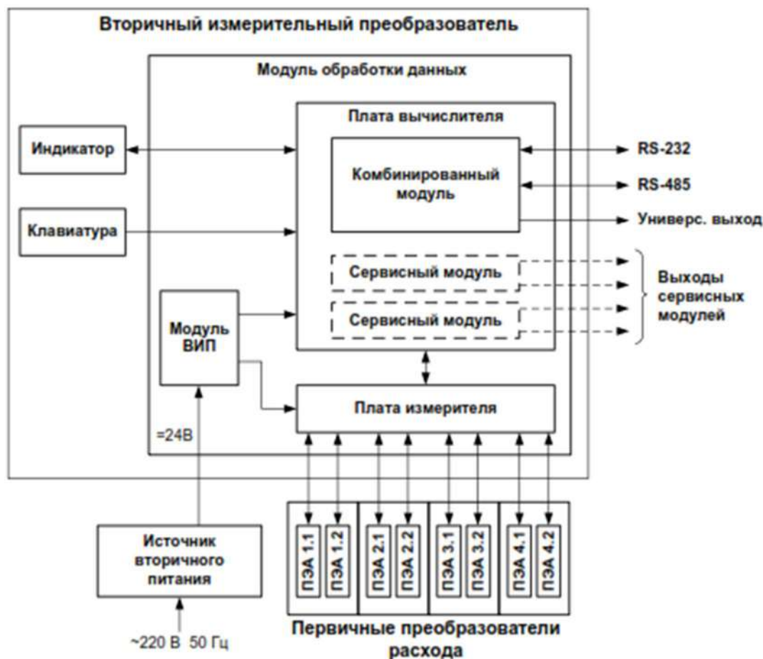
Рисунок 3 – Структурная схема расходомера
