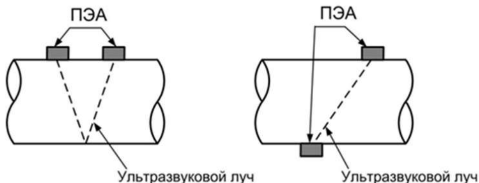
Рисунок 2 – Схемы установки ПЭА на трубопроводе
