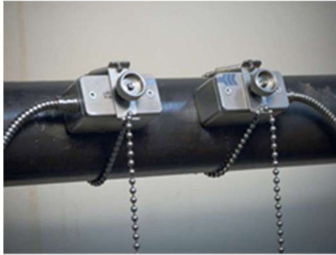
Рисунок 23- Накладные датчики (ПЭП)
